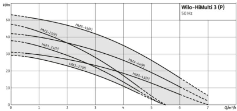
Charakterystyka Wilo HiMulti3
