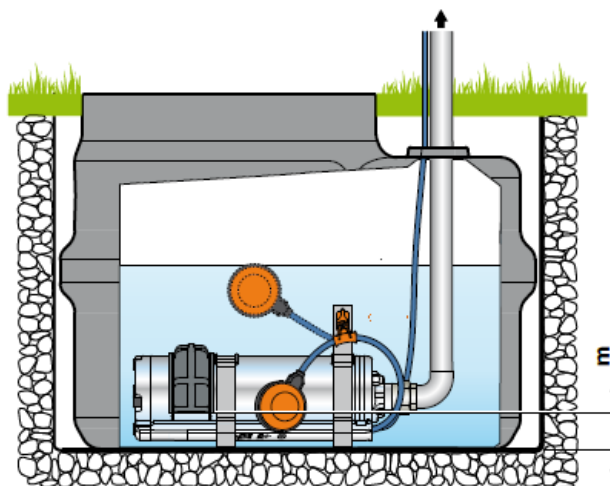
Typ montażu w poziomie
