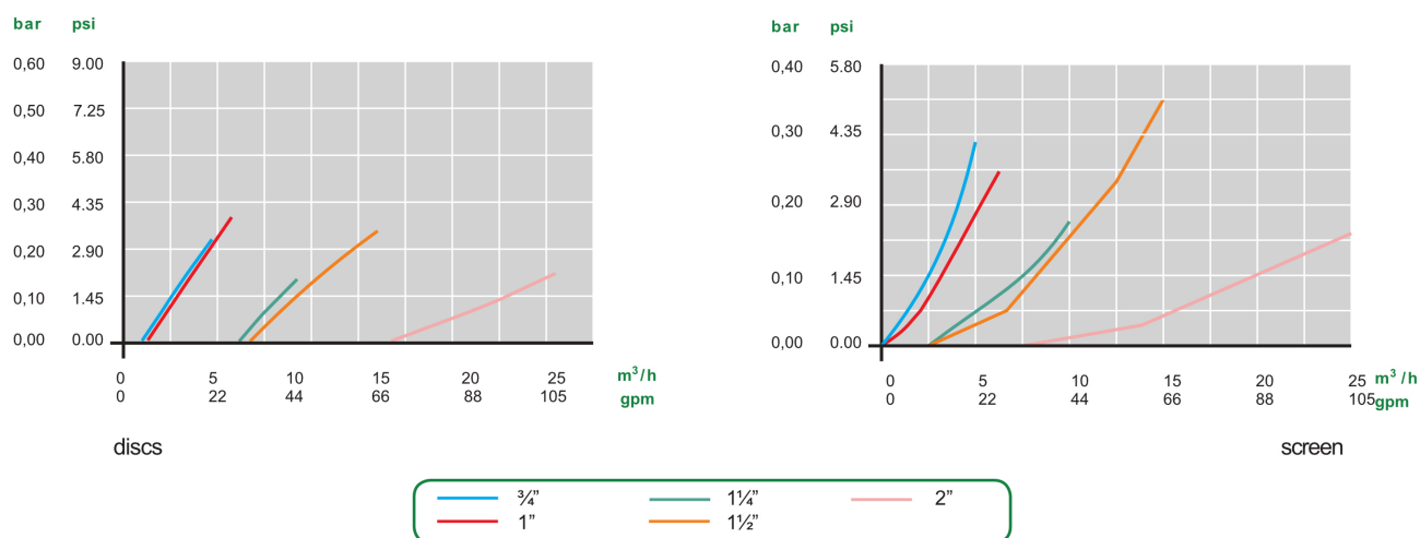
Wykres strat ciśnienia na filtrach Cepex:
