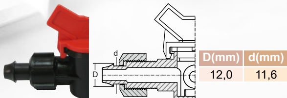
Offtake Πιπέτα
