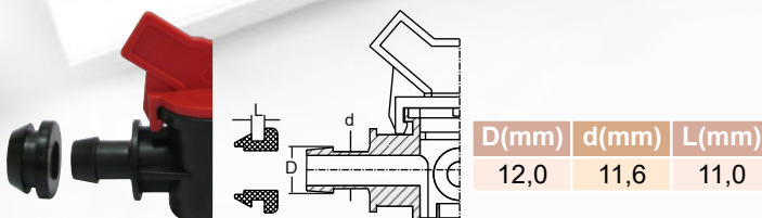
Grommet Γρόμετ
