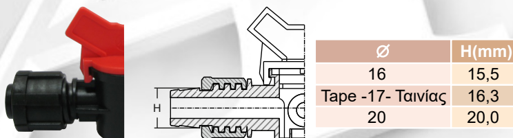
Dripper pipe - Tape Σταλακτηφόρου σωλήνα - Ταινίας
