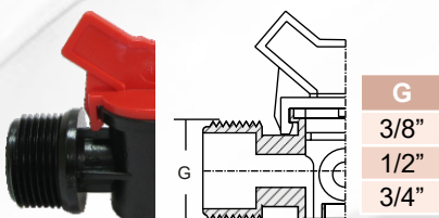
Nipple Male threaded Νίπελ Αρσενικό
