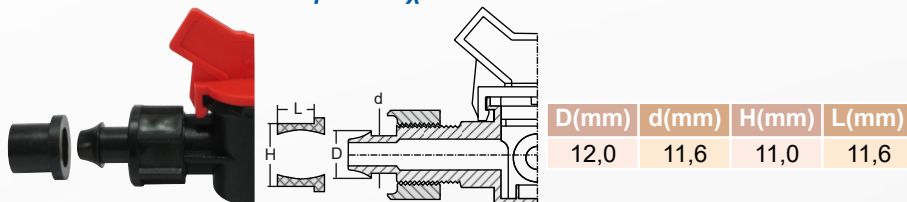
Offtake with rubber Πιπέτα με λάστιχο
