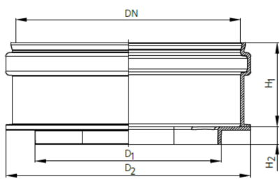
Wymiary
