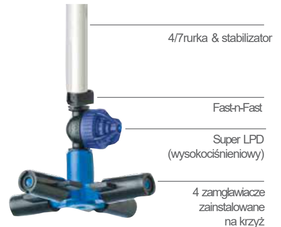
PRZEŁYWZAMGŁAWIACZA KRZYŻOWEGO ( l/h )
