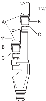
Рис. 3 Ежектор з пластмасовим трубним з'єднанням
