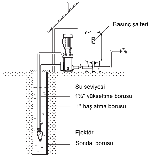
Şekil 2 Derin kuyu pompalı pompa sistemi
