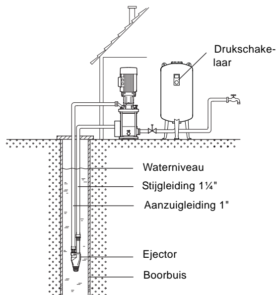
Afb. 2 Pompsysteem met pomp voor diepe putten
