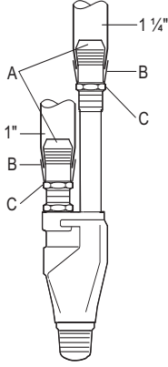
Şekil 3 Plastik tüp bağlantılı ejektör
