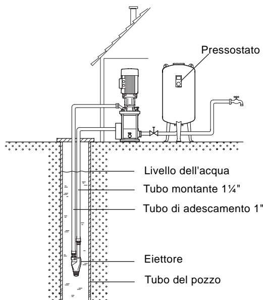
Fig. 2 Impianto di pompaggio con pompa per pozzo profondo
